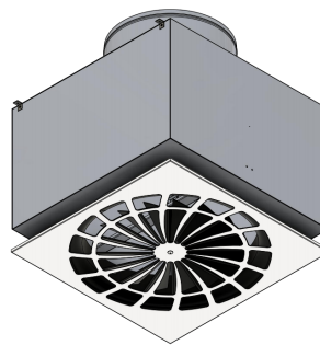
Connexion verticale
