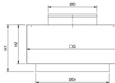
Raccordement vertical (sortie opposée)
