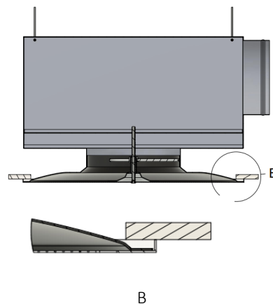
Montage en faux plafond continu
